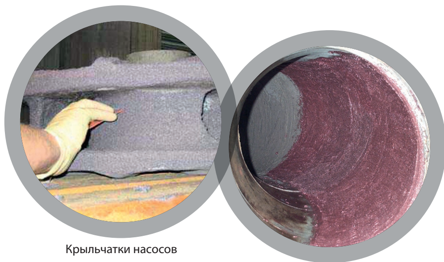
Отводы труб
