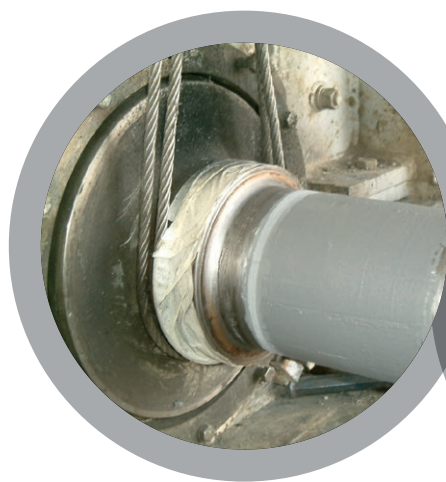
Восстановление вала
