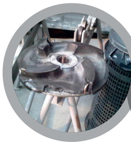
Крыльчатки насосов
