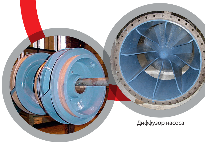
Крыльчатки насосов
