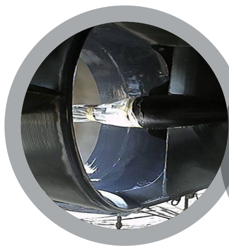
Насадки Корта
